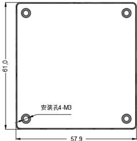
标准型 61.0*57.9*12.7mm
