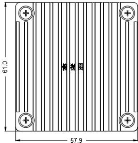
标准型+散热器 61.0*57.9*27.7mm
