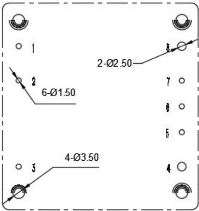
推荐PCB开槽尺寸
